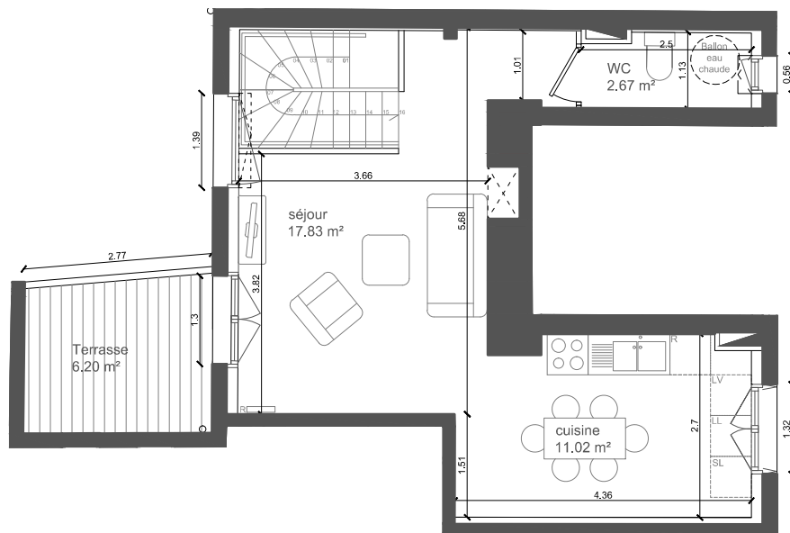
NIVEAU R+2
