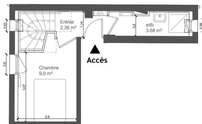
NIVEAU R+1
